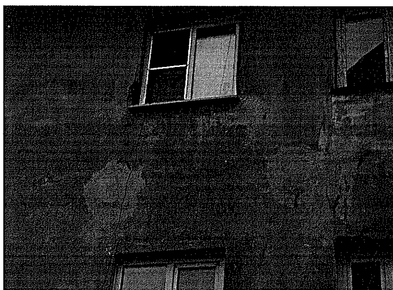
Рис. 1, 2, 3 Фрагменты западного фасада. Разрушения кирпичной кладки, отслоения штукатурного и окрасочного слоев.
