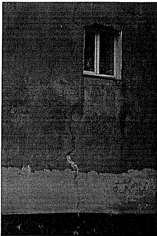
Рис. 4 Фрагмент торцевого южного фасада. Вертикальная трещина, разрушение перемычки.
